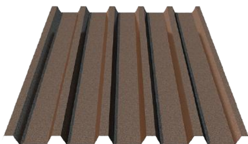
Профилированный лист МП-20х1100-А Толщина материала: 0,4–0,8 мм
